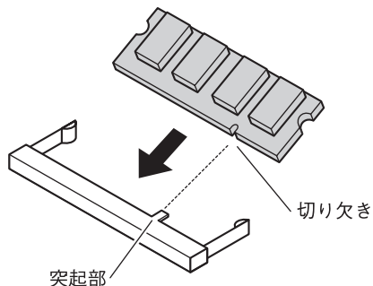
突起部と切り欠きの位置はイラストと異なる場合があります。
