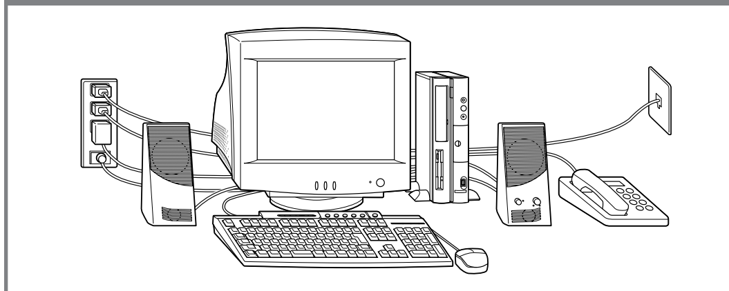
接続完成図(前面)
